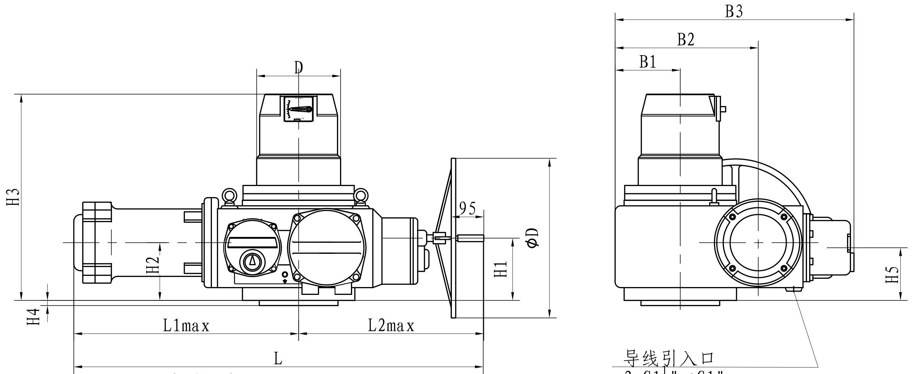
SCD-3、4外形尺寸图
